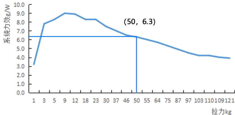
拉力-系统力效
