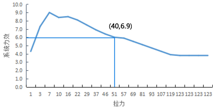
拉力-系统力效
